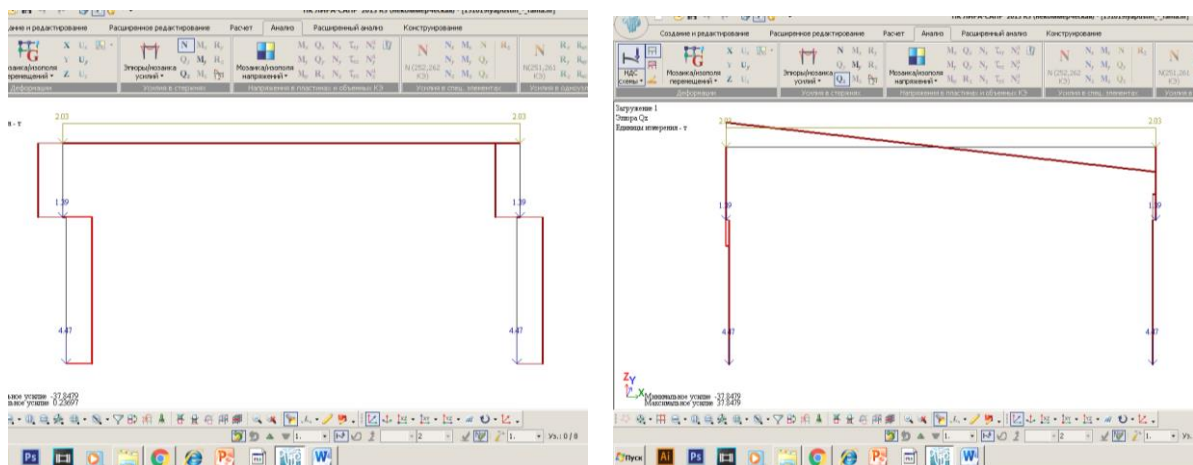
Рисунок 5. Эпюры поперечных сил и продольных сил
